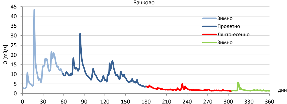
Фиг. 26. Хидрограф на среднодневния отток към ХМС № 72460
