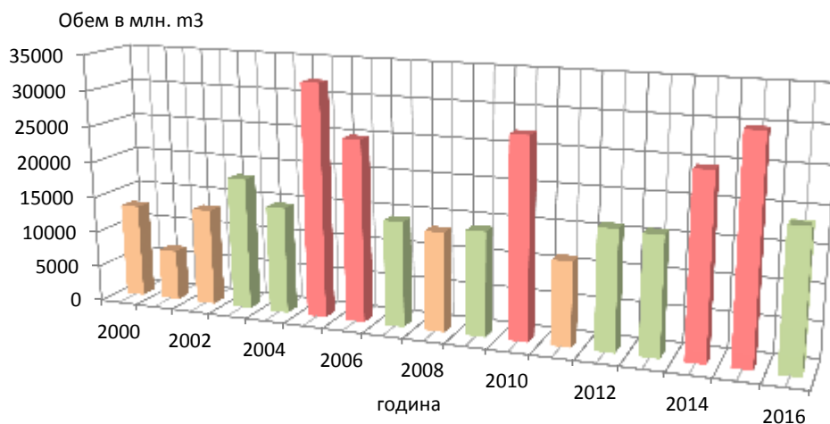
Фиг. 21. Годишен обем на повърхностния отток за периода 2000 ÷ 2016 г.
