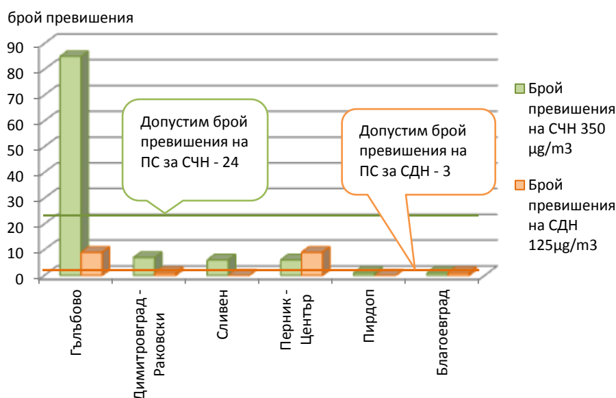
Фиг. 17. Превишения на нормите за SO 2 за 2016 г.
