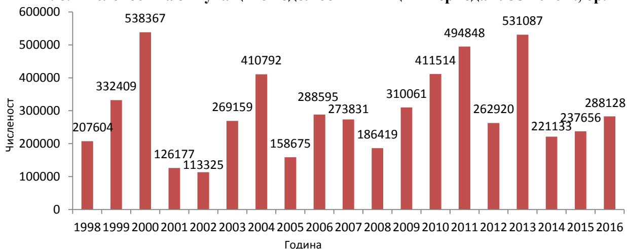
Фиг. 6. Численост на зимуващите водолюбивии птици в периода 1998-2016 г., бр.
