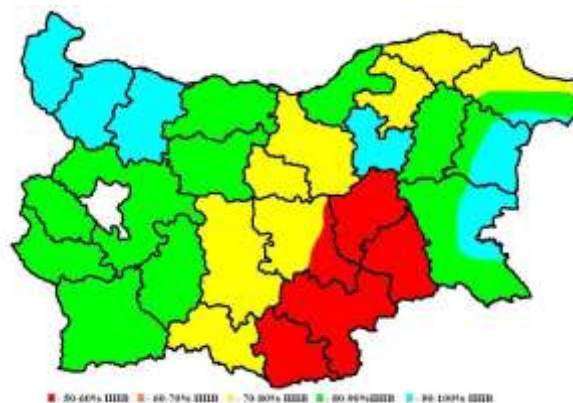
Фиг. 7. Пространствено разпределение на водните запаси в почвите на 27.10.2016 г. в еднометровия почвен слой (% от ППВ)*
