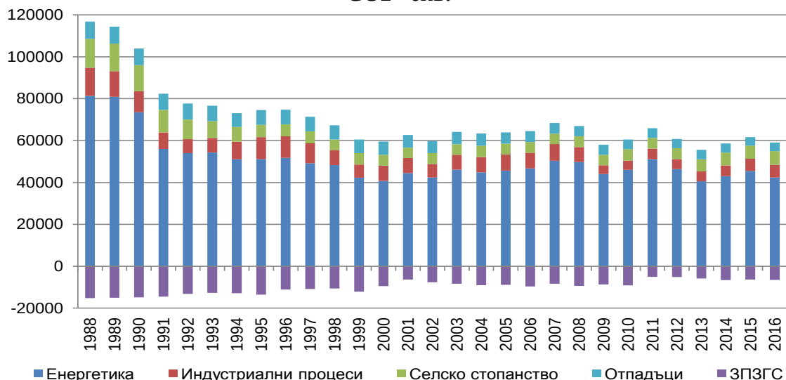
Фиг. 12. Общи емисии на парникови газове по сектори за периода 1988 – 2016 г., Gg CO 2 - екв.
