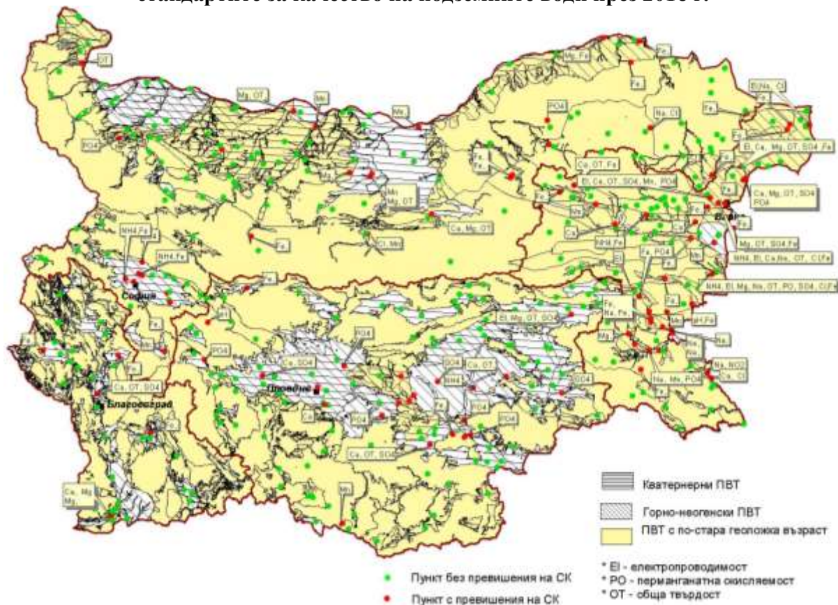
Фиг. 33. Подземни водни тела и мониторингови пунктове с показатели над стандартите за качество на подземните води през 2016 г.
