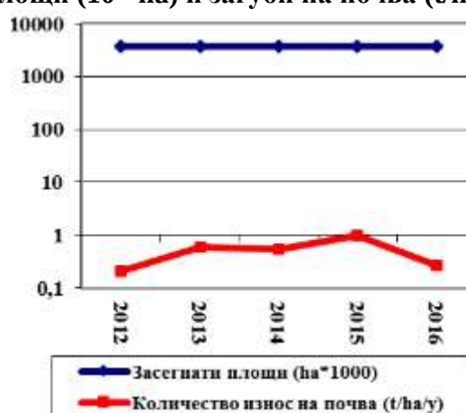
Фиг.19. Тенденции в разпределението на ветровата ерозия в страната. Засегнати площи ( 10^3 ha) и загуби на почва (t/ha/y)
