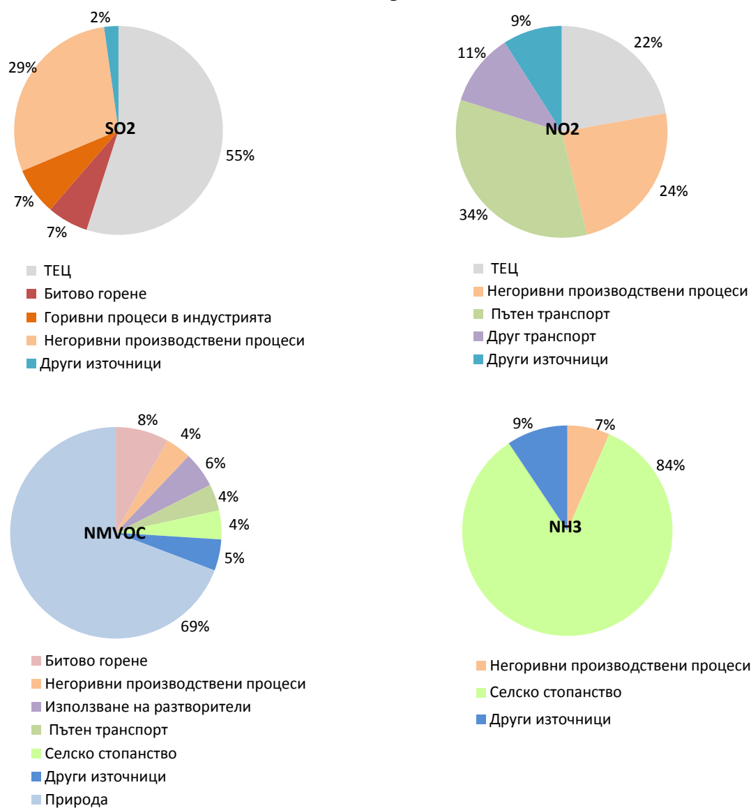
Фиг.3. Разпределение на дела на емисиите на вредни вещества по основните групи източници през 2016 г., %
