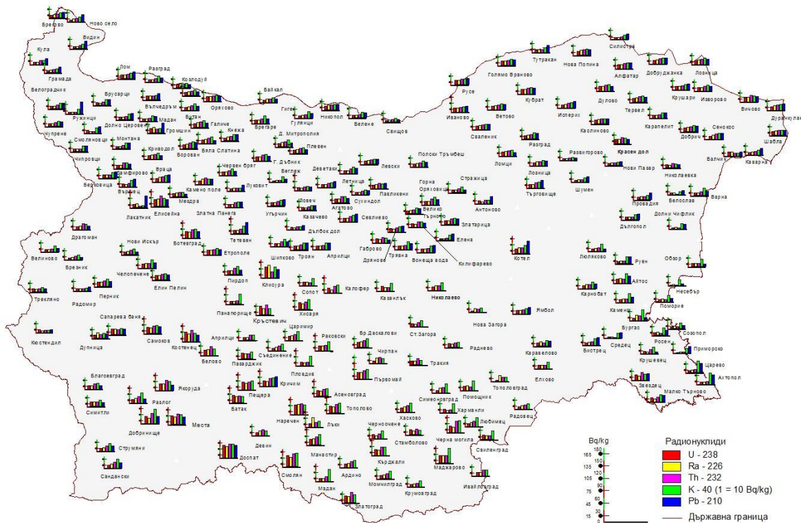
Фиг.4. Специфична активност на естествени радионуклиди в необработваеми почви, Bq/kg
