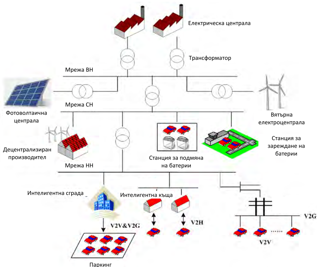
Фигура 2.30: Електрическа мрежа с децентрализирано производство на енергия и захранване на електромобили
