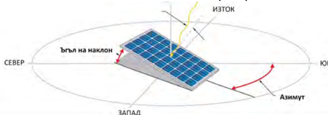
Фигура 2.4: Азимут (ориентация) и ъгъл на наклон
