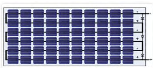
Фигура 2.9: Свързване на клетките във фотоволтаичен модул
