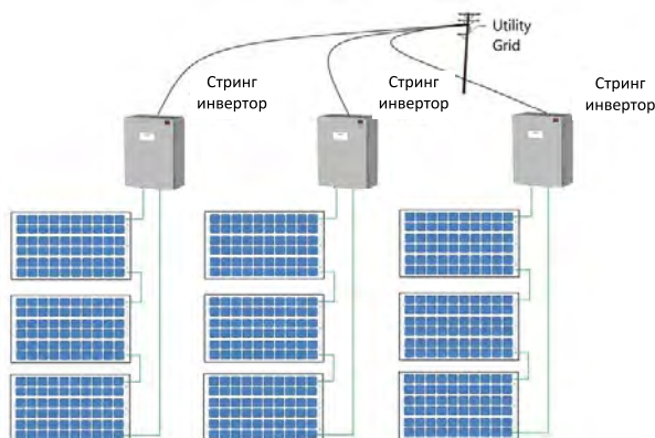
Фигура 2.21: Конфигурация на фотоволтаична система с еднострингови инвертори
