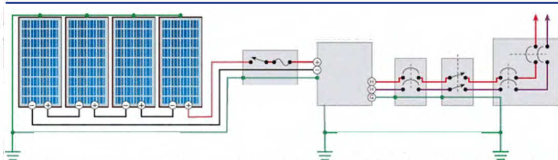
Фигура 2.19: Схема на защита от свръхнапрежение за фотоволтаична система с прекъсвачи
