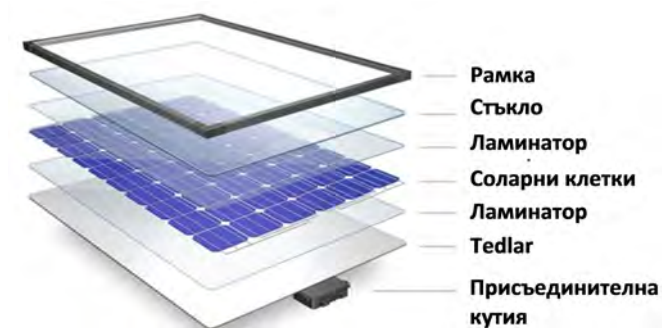
Фигура 2.8: Основни компоненти на фотоволтаичния модул
